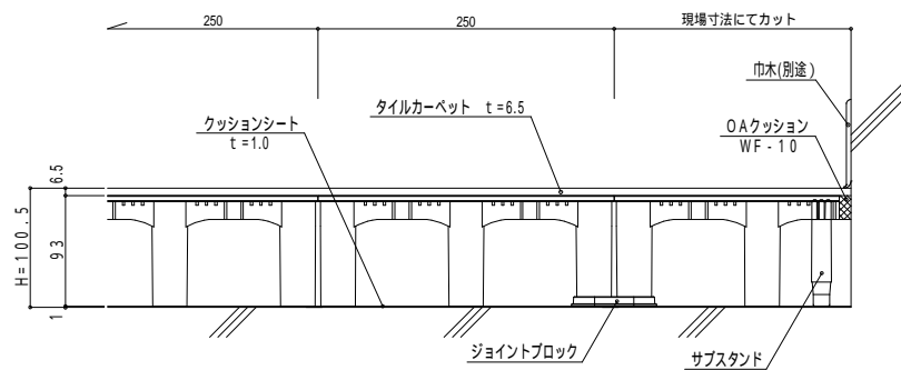
断面図 S = 1 : 5
